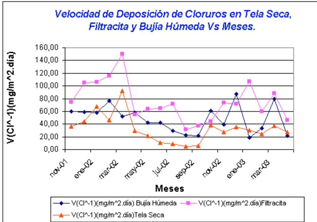
Fig. 1: Velocidad de deposición de cloruros determinados en diferentes captadores.
