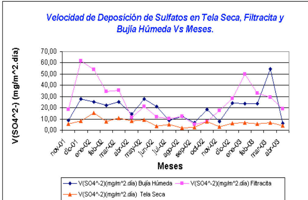
Fig. 2: Velocidad de deposición de sulfatos determinados en diferentes captadores. ANEXO 5.
