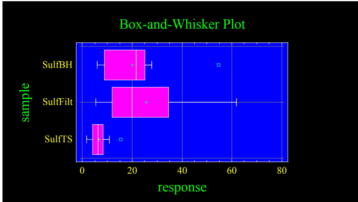
Fig. 6: Gráfico Box-and-Whisker de la velocidad de deposición de iones sulfato en los captadores Bujía Húmeda, Filtracita y Tela Seca.
