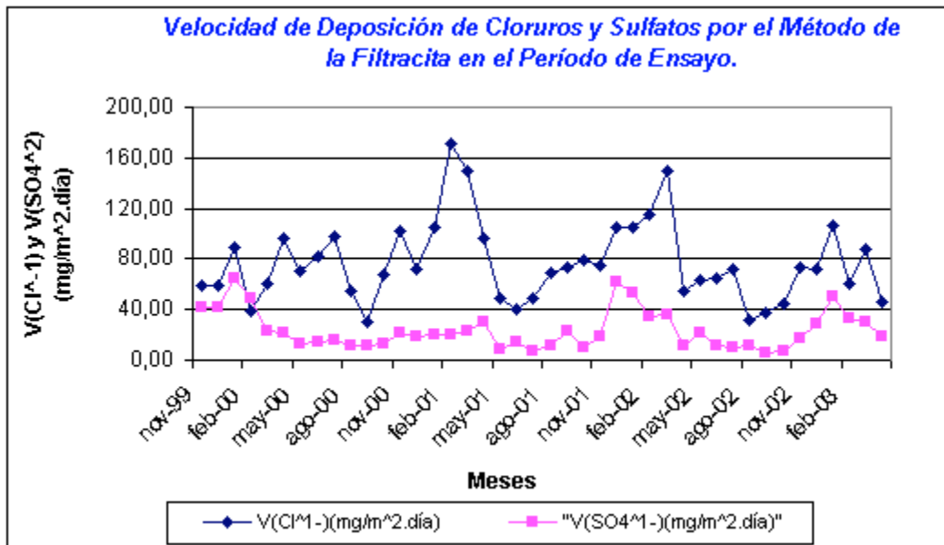
Fig.3: Velocidad de deposición de cloruros y sulfatos por el método de la Filtracita.
