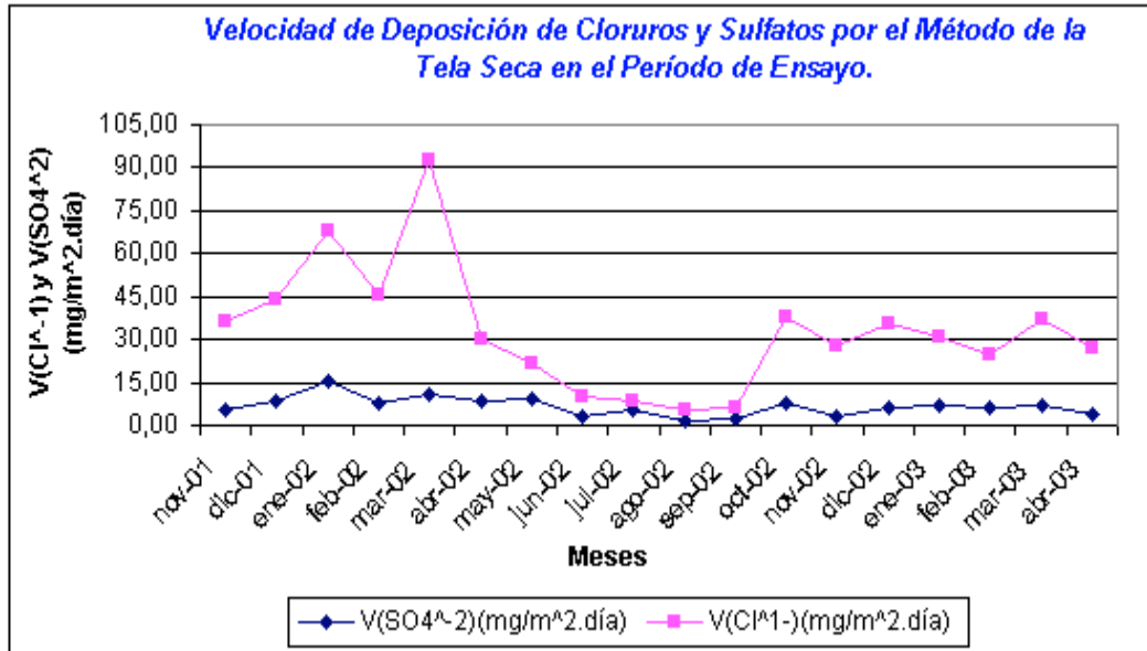
Fig.4: Velocidad de deposición de cloruros y sulfatos por el método de la Tela Seca.
